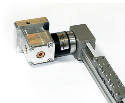
Version mit Planetengetriebe
