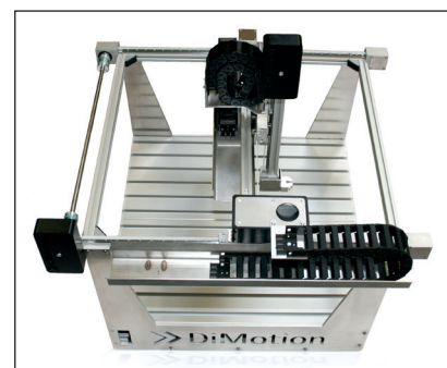
Portalversion inkl. möglichem Anbau von Servo- oder Schrittmotoren
