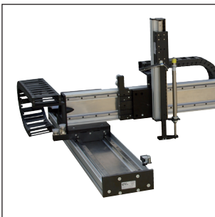
3-Achs-Ausleger-Flächen- portal mit Grundachse MLE5, Ausleger MLE3 und Vertikal- achse MLU3
