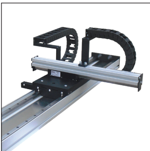
2-Achs-Ausleger-Portal mit Grundachse MLE5 und Querachse MLU3
