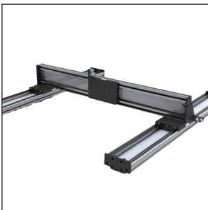
2-Achs-Portal mit zwei parallelen Grundachsen MLE3 und Querachse MLE5
