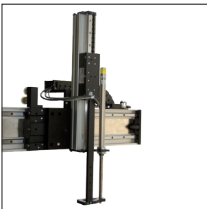
2-Achs-Linienportal mit Grundachse MLE3 und Vertikalachse MLU3
